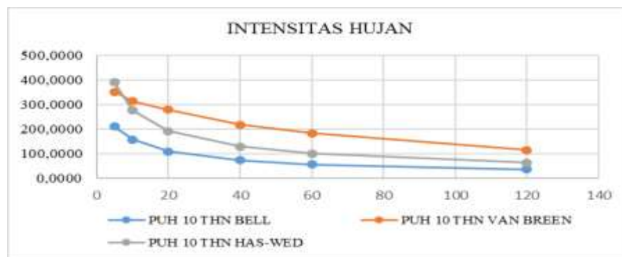
Gambar 1. Grafik Intensitas Hujan
